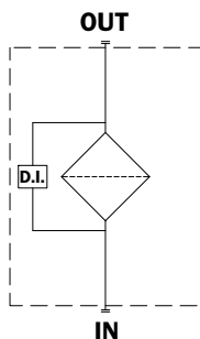
Filtro senza valvola di bypass
