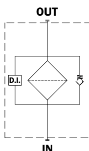
Filtro con valvola di bypass
