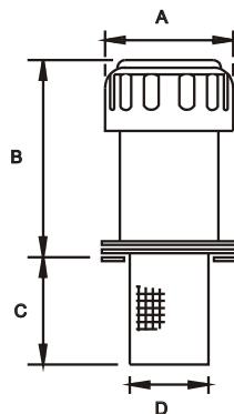
FSB-25 HN
